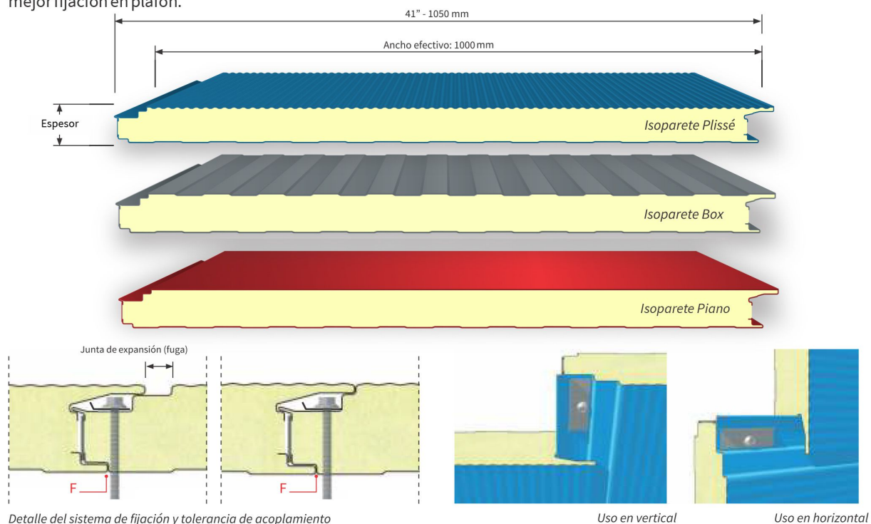
Detalle del sistema de fijación y tolerancia de acoplamiento
